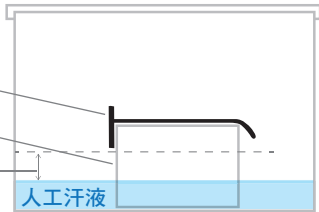
圖：抗汗液腐蝕測試儀器簡圖。
